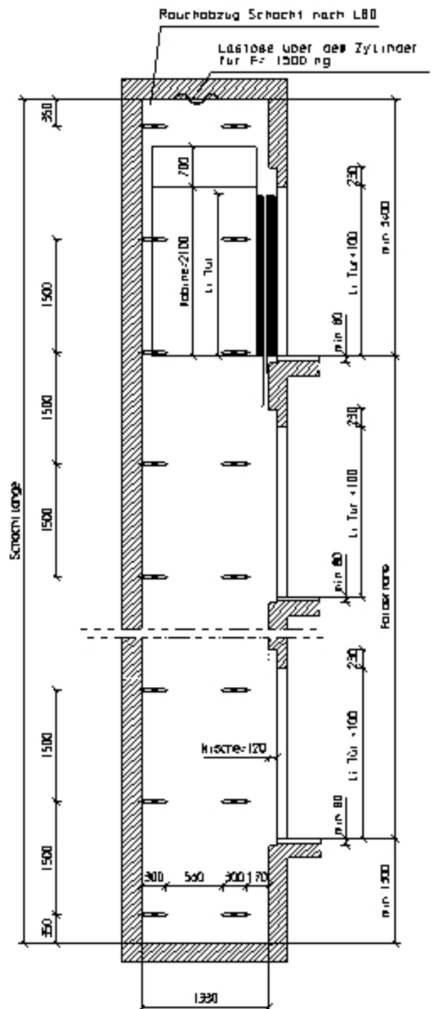
Schnitt A-A
