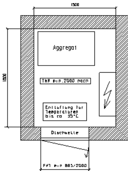
Triebwerksraumgrundriß
