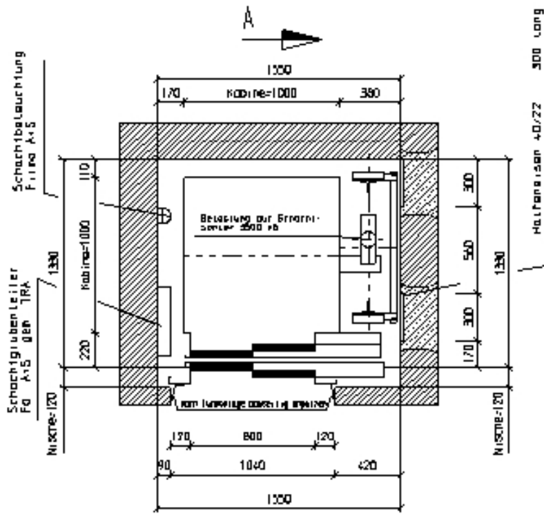
Schachtgrundriß
